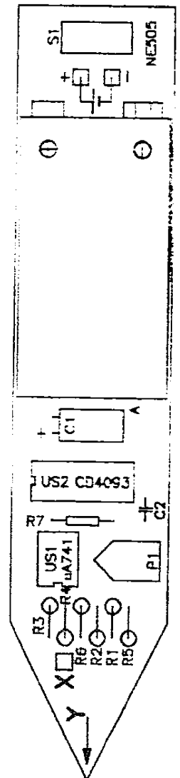
Schemat montażowy
