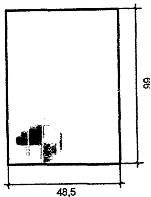
WYMIARY OBUDOWY KM 62
